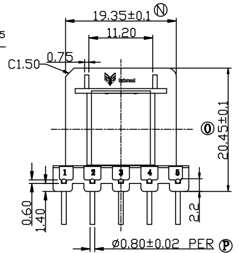
SEC:B-B
