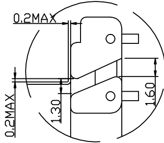
D部放大图 2:1
