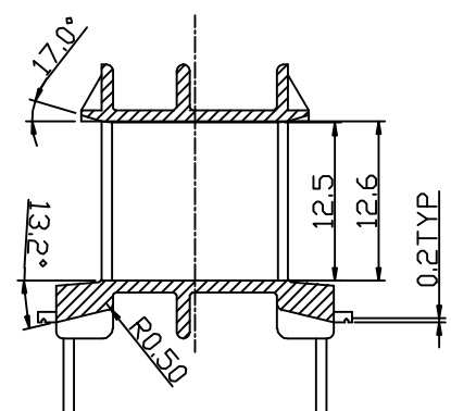
SEC:B-B
